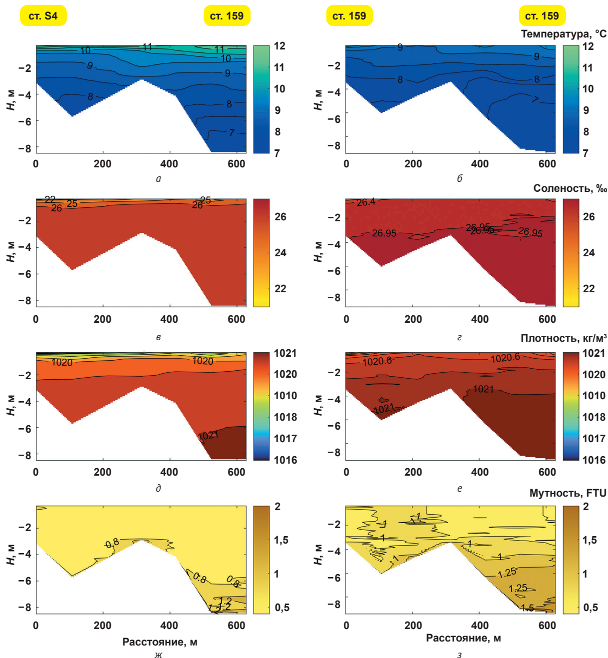
Рис. 3. Распределение температуры (а, б), солёности (в, г), плотности (д, е) и мутности (ж, з) воды на отливе (левые панели) и приливе (правые панели) 16 июня 2025 г.
